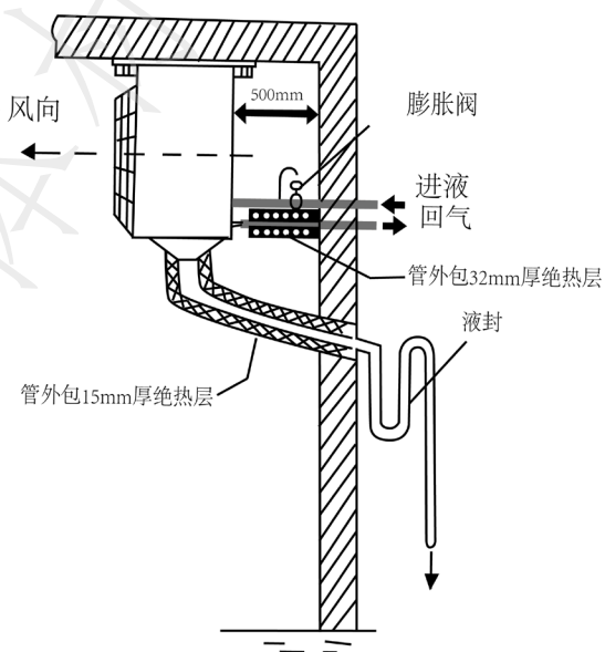
图1 冷风机安装示意图
